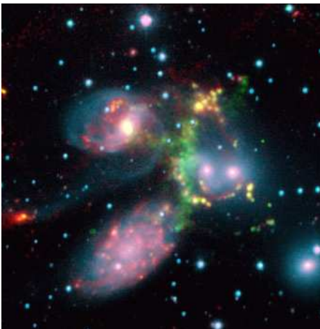
Abb 1.: Dieses Falschfarben-Komposit der Zentralregion des Stephans Quintett zeigt ein kompliziertes Geflecht aus Galaxien und intergalaktischem Medium. Das Muster entstand durch die Wechselwirkung der Galaxie NGC7318b (blaue Wolke rechts der Mitte) mit ihrer Umgebung: Das Milchstraßensystem rast mit einer Geschwindigkeit von 1000 Kilometern pro Sekunde in das intergalaktische Medium und erzeugt dadurch eine Schockwelle, die im Licht von Wasserstoffmolekülen grün leuchtet. Das Bild entstand durch die Überlagerung von Aufnahmen, die mit dem Observatorium auf dem Calar Alto in Spanien und dem Weltraumteleskop Spitzer gewonnen wurden. Bild: NASA/JPL-Caltech
