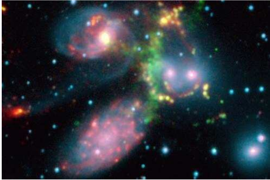
Falschfarben-Bild: Eine Galaxie (blaue Wolke) erzeugt eine Schockwelle, die im Licht von Wasserstoffmolekülen grün leuchtet. (Bild: Nasa/JPL-Caltech)
